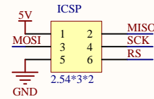
ICSP Header
